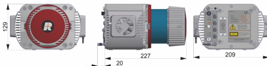
前视图
